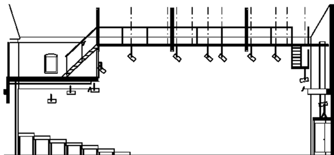
Vic SECCO F-F vista general de Escala 1:100
